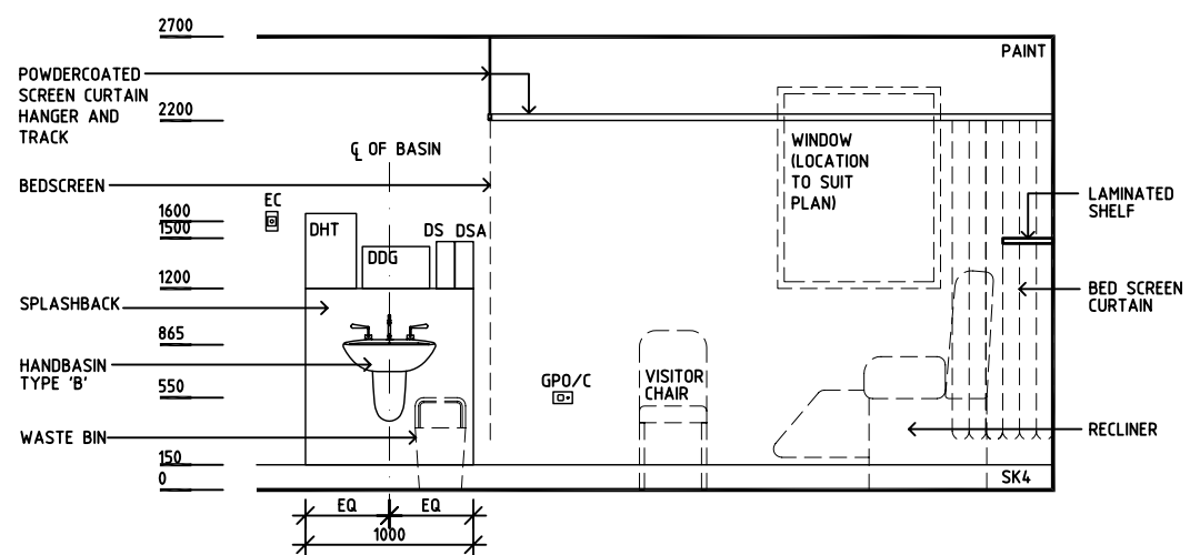
ELEVATION 2
