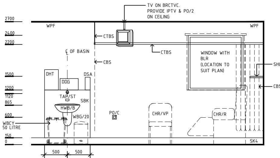
ELEVATION 2
