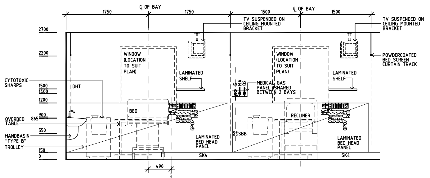
ELEVATION 1
