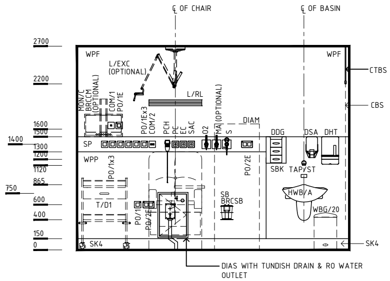
ELEVATION 2
