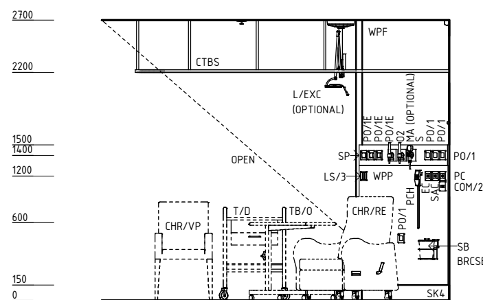
ELEVATION 02
