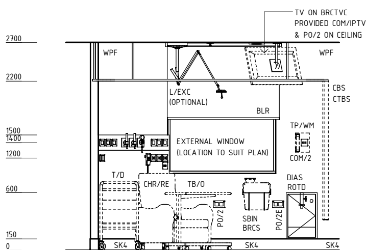
ELEVATION 01
