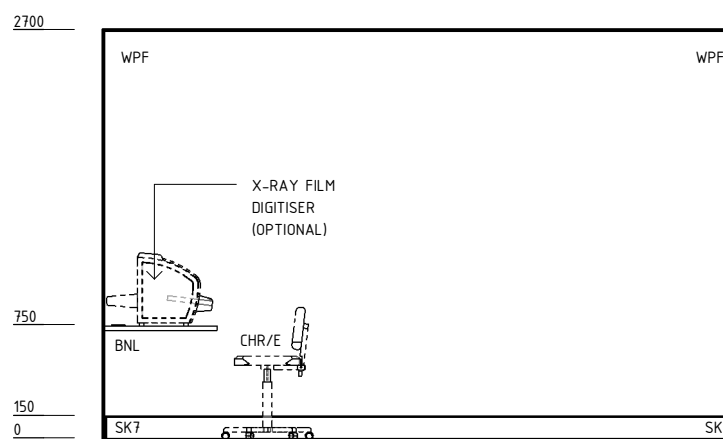
ELEVATION 2
