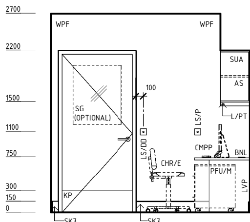
ELEVATION 3
