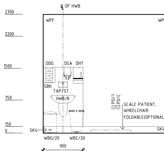
ELEVATION 2
