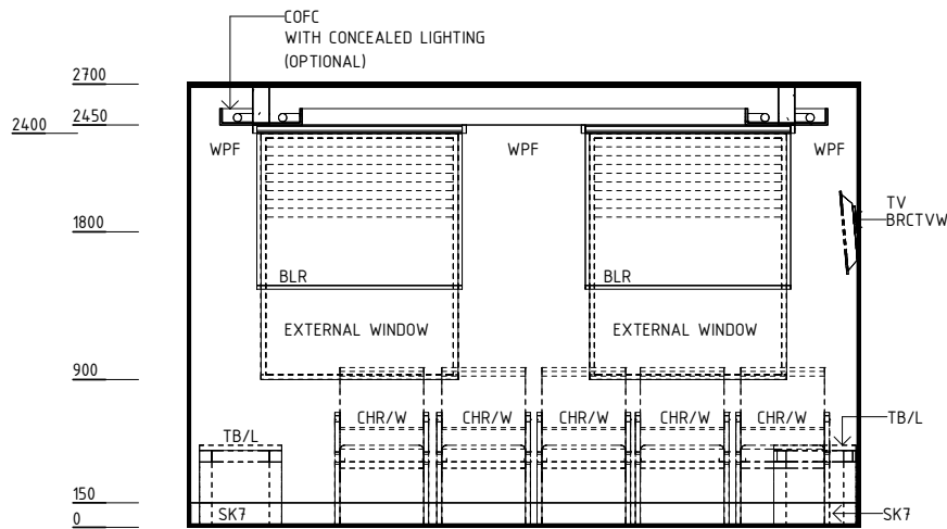
ELEVATION 1
