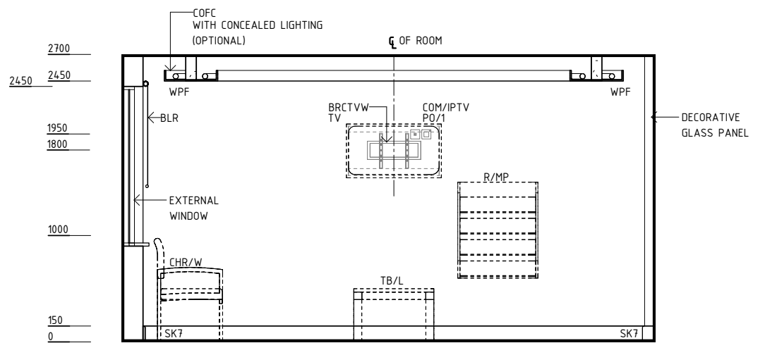
ELEVATION 2
