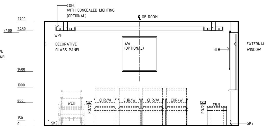
ELEVATION 4
