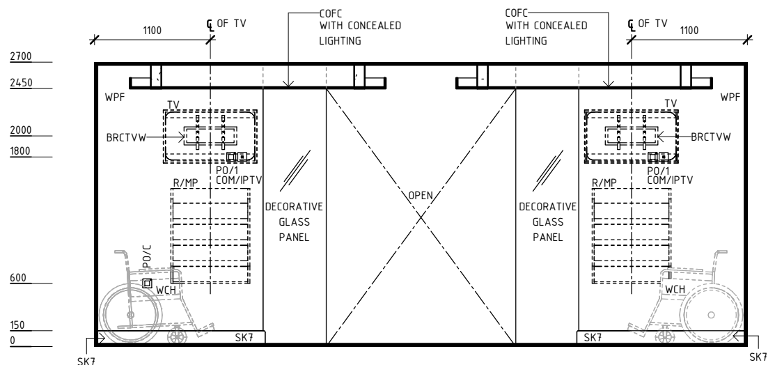
ELEVATION 3
