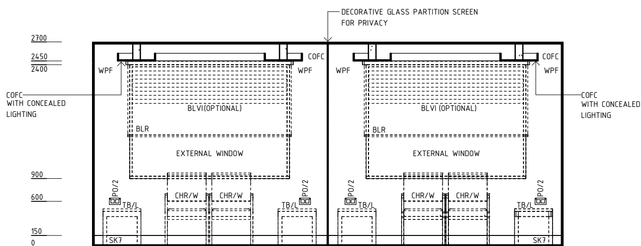
ELEVATION 1
