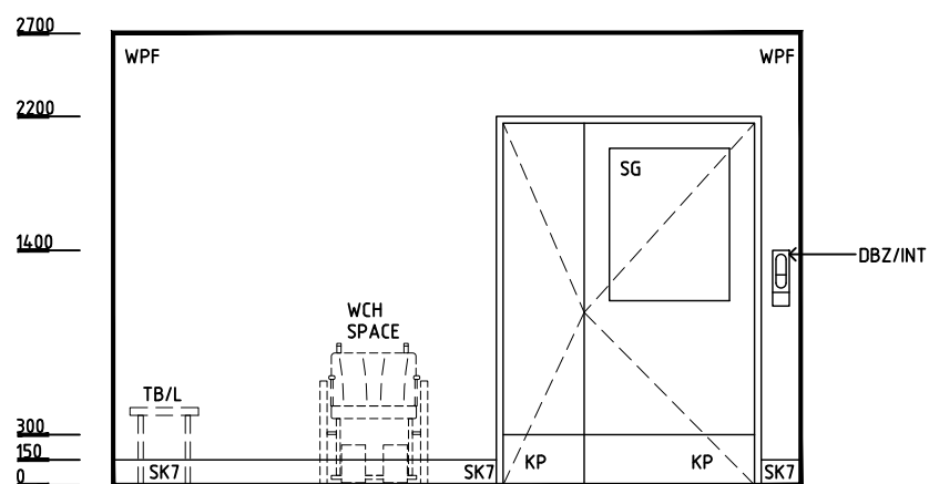
ELEVATION 1
