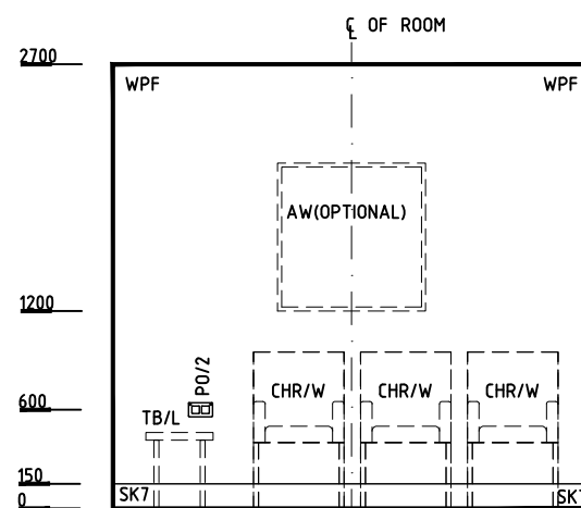
ELEVATION 4
