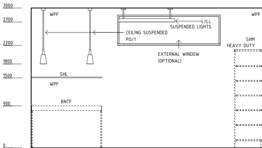
ELEVATION 1
