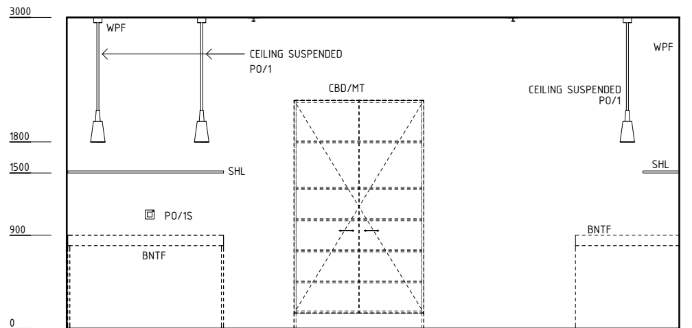
ELEVATION 4
