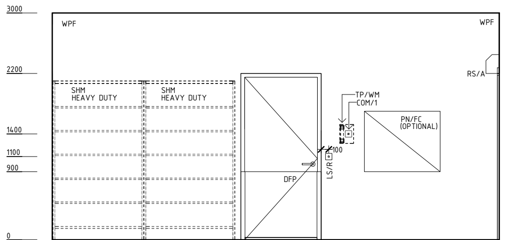
ELEVATION 2
