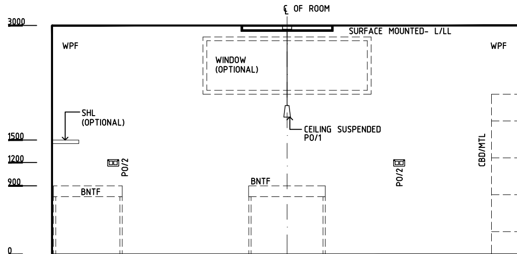
ELEVATION 1
