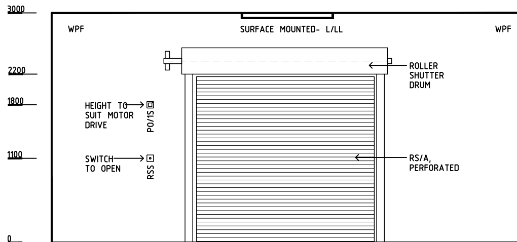
ELEVATION 3
