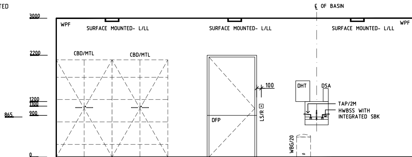
ELEVATION 2
