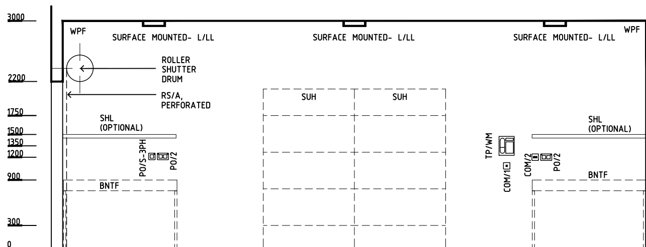
ELEVATION 4
