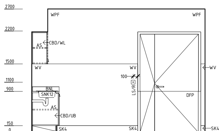
ELEVATION 3
