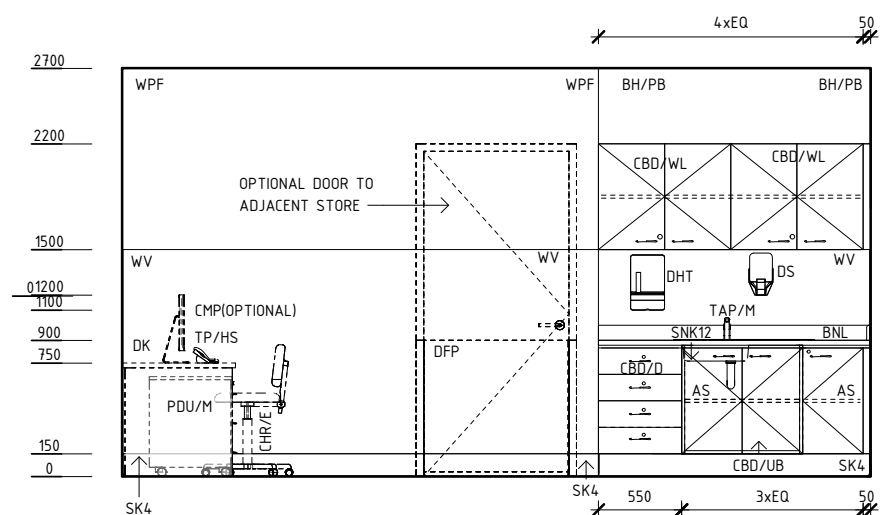
ELEVATION 2
