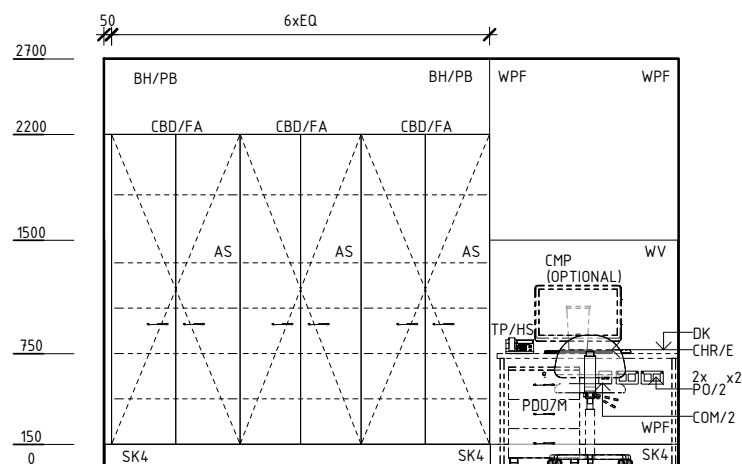
ELEVATION 1
