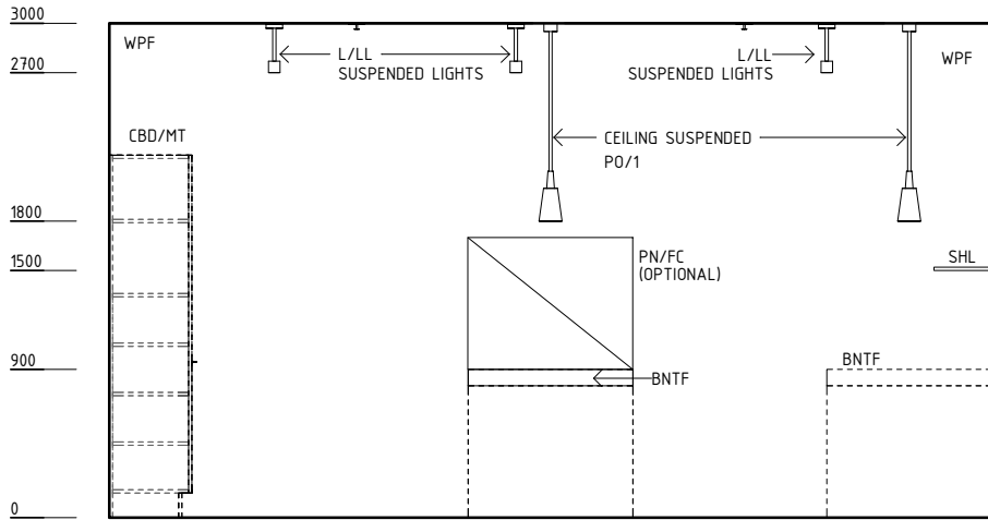
ELEVATION 4
