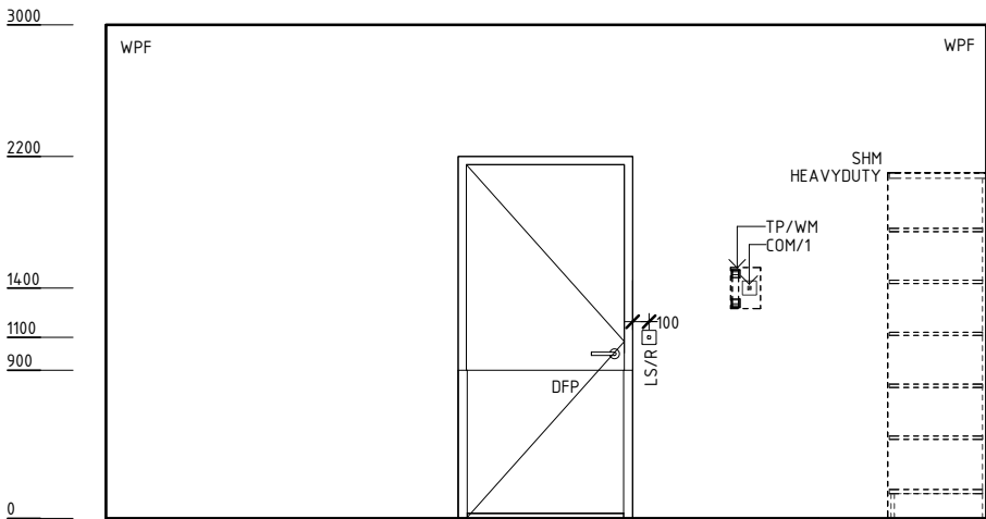
ELEVATION 2
