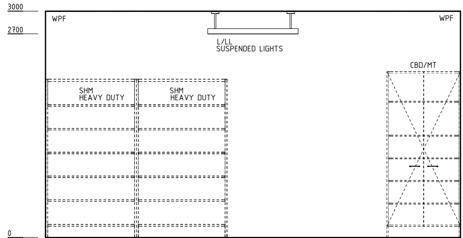
ELEVATION 3
