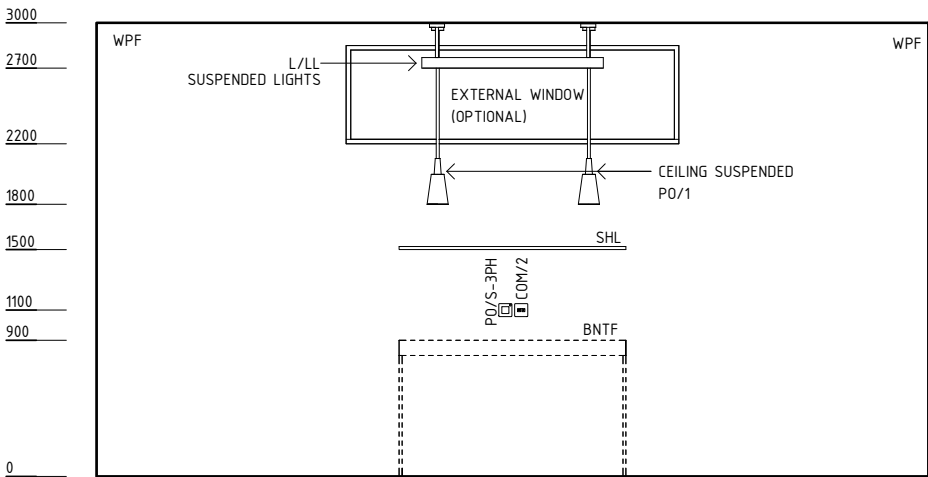
ELEVATION 1
